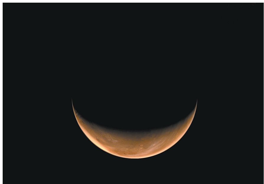
南半球上方火星影像。南半球影像由“天问一号”中分辨率相机于北京时间2021年3月16日拍摄,此时环绕器轨道高度约1.12万千米。3月26日,国家航天局发布2幅由我国首次火星探测任务“天问一号”探测器拍摄的南、北半球火星侧身影像。图像中,火星呈“月牙”状,表面纹理清晰。新华社发(国家航天局供图)
