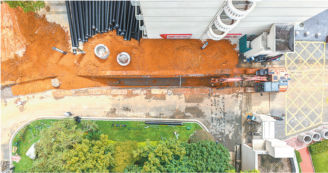
近日，赣县区城南片区排水防涝和雨污分流设施改造提升项目一标段施工现场，工人在铺设地下管网。项目建成后，将有效解决城南片区污水排放不畅和城北片区雨水排水问题，污水收集率预计提升至75%，惠及城区数十万居民。
