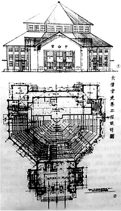
赣闽师院大礼堂(中山堂)设计1正立面图2一层、二层平面图。(资料图片)
